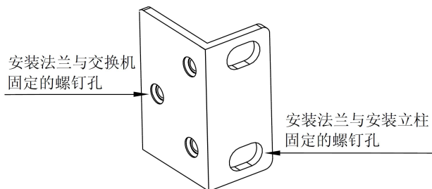
图 13. 安装法兰
