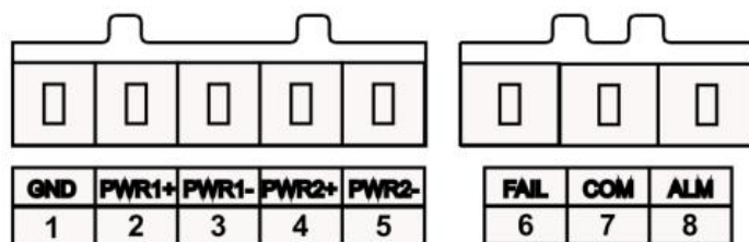
图 11. 电源、告警连接端子布置图
